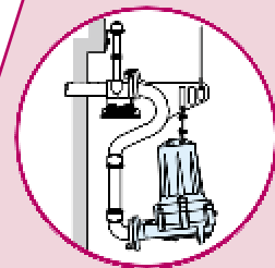
Ovješena automatska spojka
