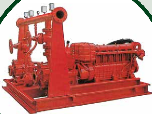
Moto-pumpa za gašenje požara
